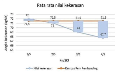
Gambar 10. Grafik Hasil Pengujian Kekerasan Kuningan/Serbuk Kayu Jati (SKJ)
