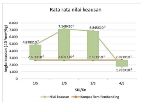
Gambar 14. Grafik Hasil Pengujian Keausan Serbuk Kayu Jati (SKJ)/Kuningan
