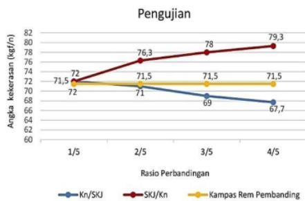
Gambar 12. Grafik Hubungan Hasil Pengujian Kekerasan
