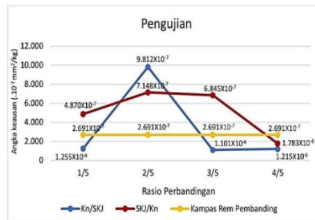
Gambar 15. Grafik Hubungan Hasil Pengujian Keausan
