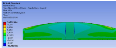
Gambar 47. Tegangan normal serat kaca pada sayap drone Airawata
