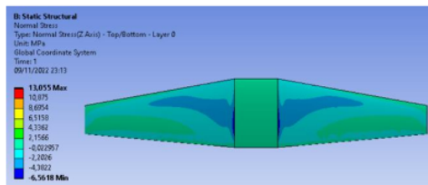
Gambar 50. Tegangan normal serat kaca pada sayap drone baru
