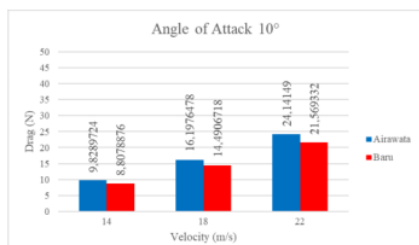
Gambar 36. Grafik perbandingan gaya hambat pada kondisi sudut serang 10°
