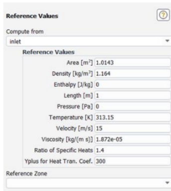
Gambar 10. Parameter pemodelan
