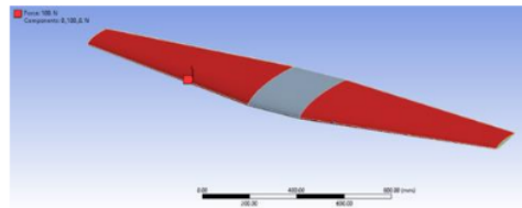
Gambar 17. Permukaan pembebanan
