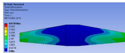
Gambar 42. Deformasi total pada sayap drone baru serat Karbon
