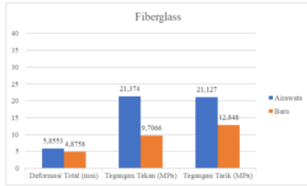
Gambar 51. Grafik perbandingan data struktur serat kaca pada drone Airwata dengan drone baru
