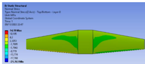
Gambar 49. Tegangan normal serat kaca pada sayap drone baru
