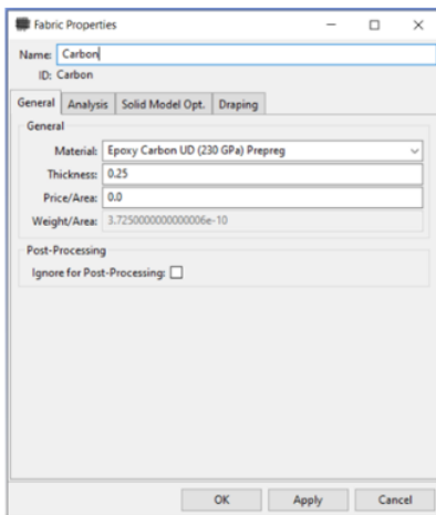
Gambar 15. Input ketebalan lapisan material
