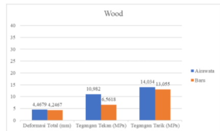
Gambar 53. Grafik perbandingan data struktur material kayu pada drone Airwata dengan drone baru
