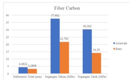
Gambar 52. Grafik perbandingan data struktur serat karbon pada drone Airwata dengan drone baru
