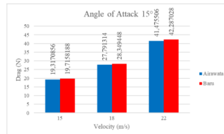
Gambar 38. Grafik perbandingan gaya hambat pada kondisi sudut serang 15°
