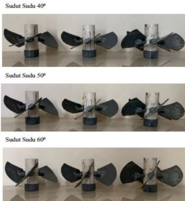
Gambar 9. Variasi Sudut Sudu
