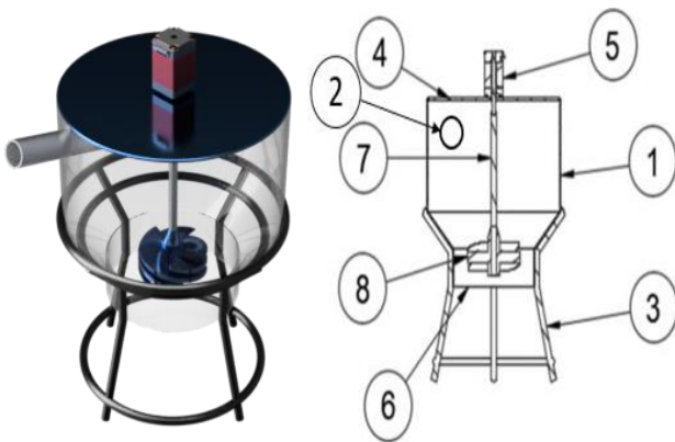
Gambar 3. Instalasi Alat
