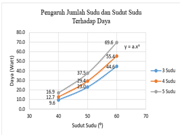
Gambar 13. Grafik Berdasarkan Daya
