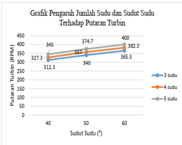
Gambar 12. Grafik Berdasarkan Putaran Turbin
