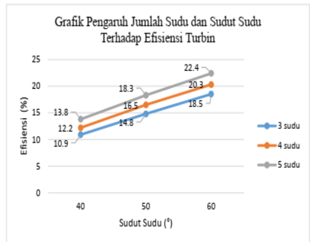
Gambar 14. Grafik Berdasarkan Efisiensi Dari Turbin
