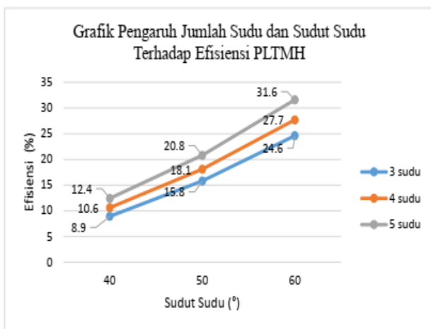
Gambar 15. Grafik Berdasarkan Efisiensi PLTMH
