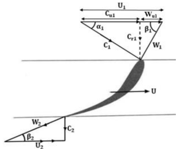
Gambar 11. Segitiga Kecepatan Turbin
