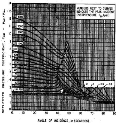
Gambar 2. Koefisien Tekanan Pantulan
