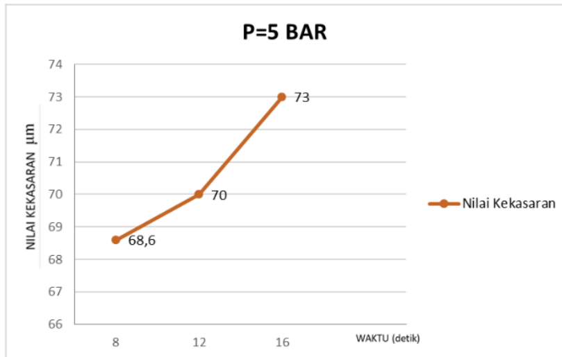
Gambar 14. grafik tekanan 5 bar dengan waktu 8, 12 dan 14 detik.
