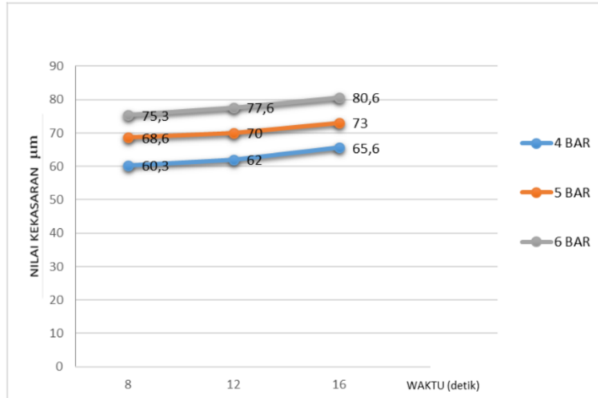
Gambar 16. Kesimpulan dari tiga grafik yang digabung menjadi satu.
