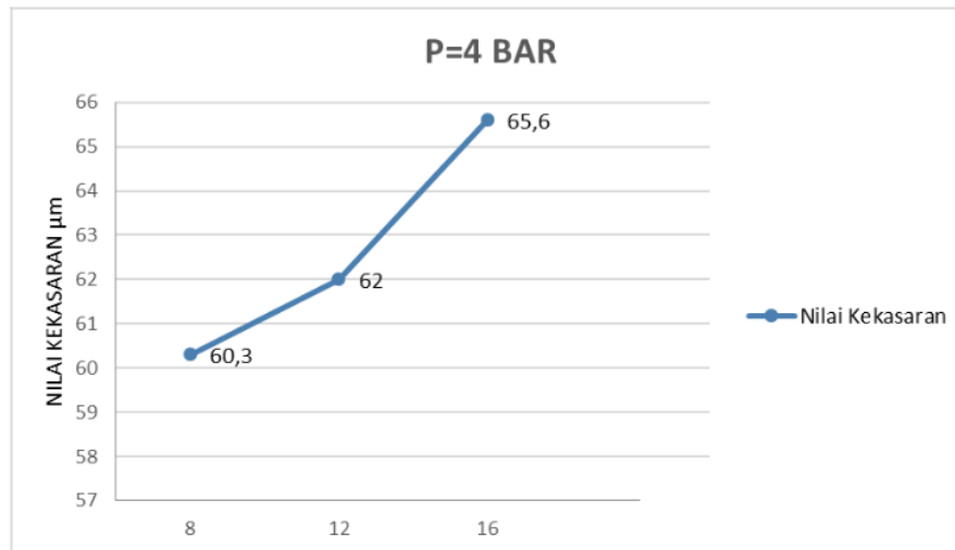
Gambar 13. Grafik tekanan 4 bar dengan waktu 8, 12 dan 16 detik.
