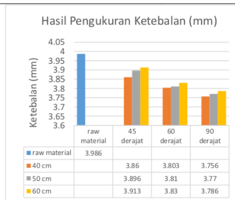
Gambar 11 Grafik hasil nilai pengukuran ketebalan
