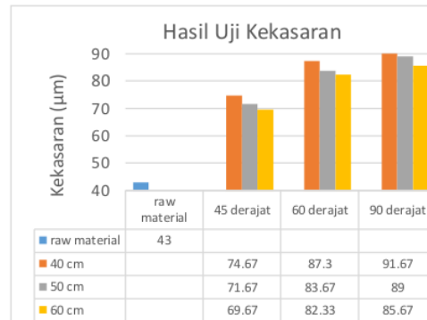
Gambar 10 Grafik nilai kekasaran
