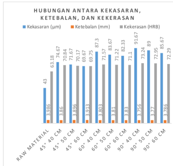
Gambar 13 Grafik hubungan antara kekasaran, ketebalan, dan kekerasan
