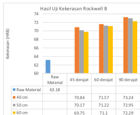
Gambar 12 Grafik hasil nilai pengukuran kekerasan
