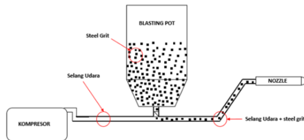
Gambar 3 Ilustrasi prinsip kerja sandblasting
