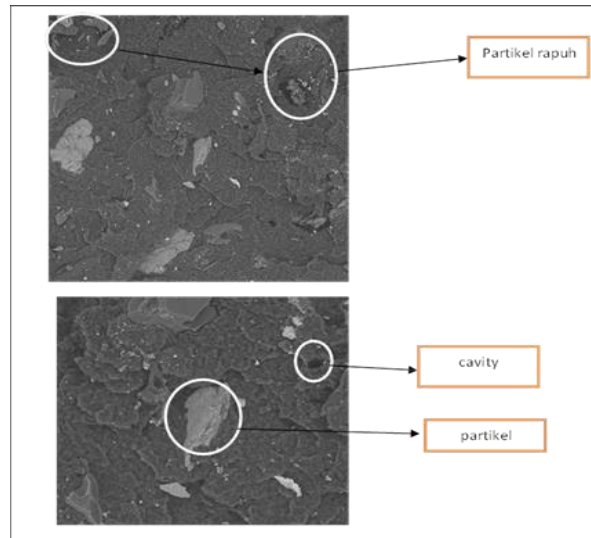
Gambar 6. Hasil Uji SEM Nilai Terendah
