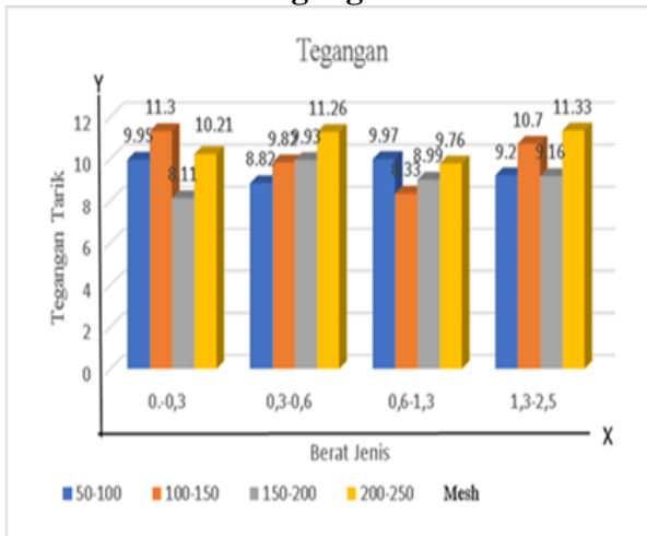
Gambarr 1. Tegangan tarik
