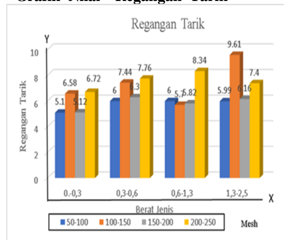
Gambar 2. Regangan tarik
