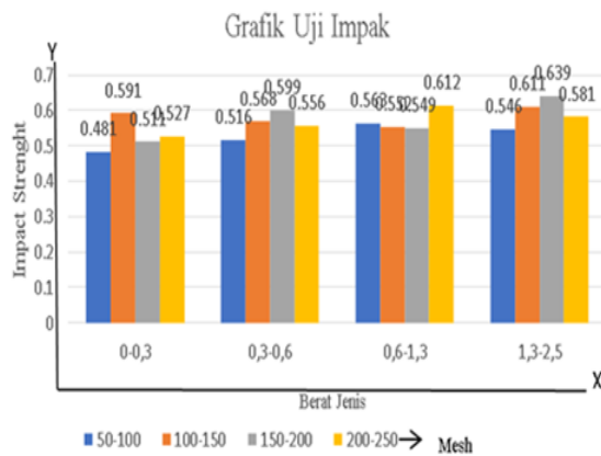
Gambar 4. Grafik Uji Impak
