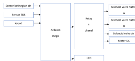
1 Gambar 3. 1 Blok.Diagram
