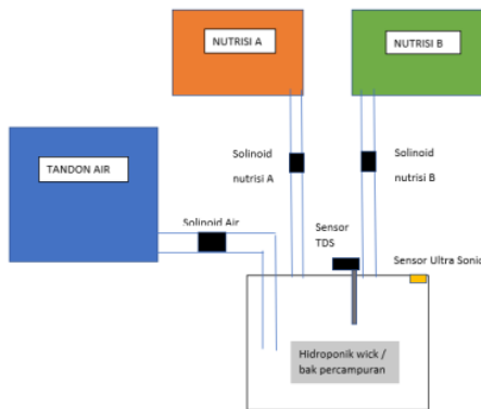
Gambar 3. 2 Desain.Mekanik
