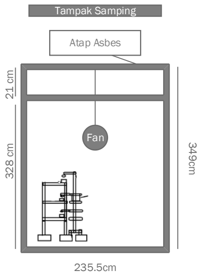
Gambar 2.9 Penempatan Alat Tampak Samping
