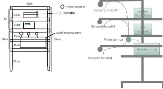
Gambar 2.5 Desain Alat
