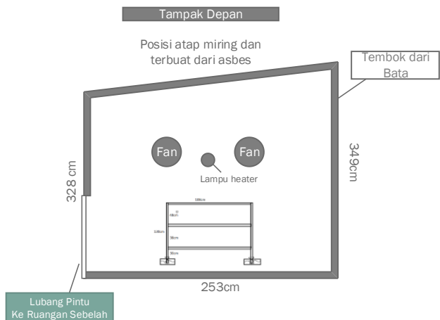
Gambar 2.8 Penempatan Alat Tampak Depan
