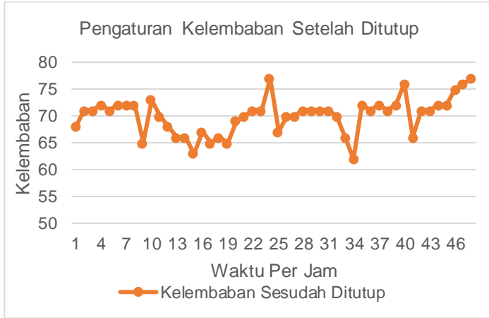
Gambar 3.7 Pengaturan Kelembaban Setelah Ditutup
