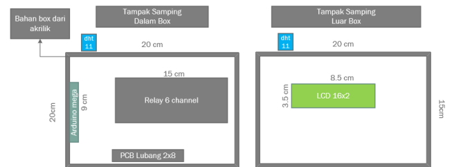
Gambar 2.3 Desain Box Kontrol Tampak Samping
