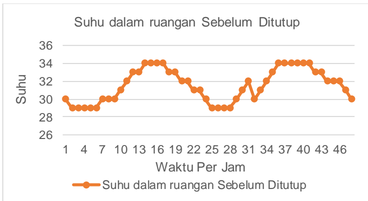
Gambar 3.2 Grafik Hasil Pengaturan Suhu
