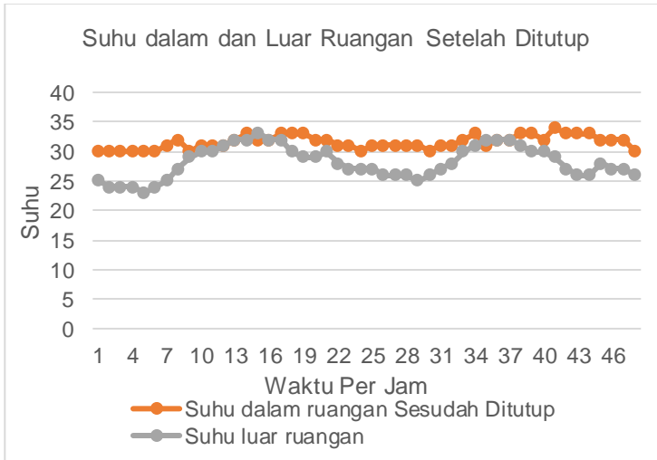
Gambar 3.8 Perbandingan Suhu Setelah Ditutup
