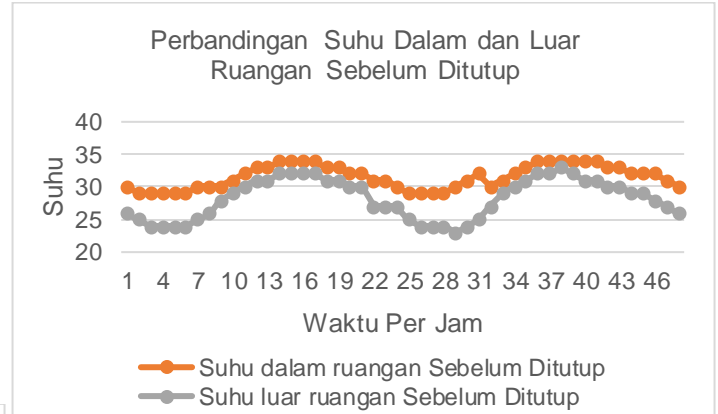
Gambar 3.4 Grafik Perbedaan Suhu
