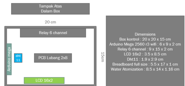
Gambar 2.4 Desain Box Kontrol tampak dari atas
