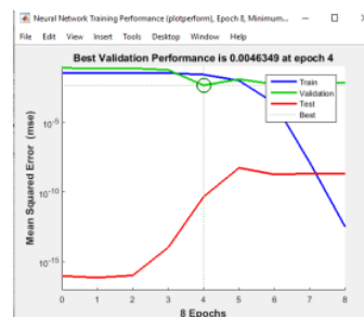
Gambar 3. Hasil validasion check terbaik JST
