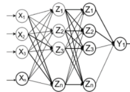
Gambar 1 Arsitektur jaringan syaraf tiruan backpropagation multilayer
