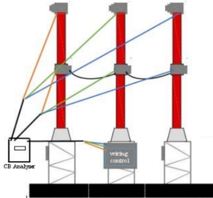
Gambar 9. Pengujian Keserampakan.
