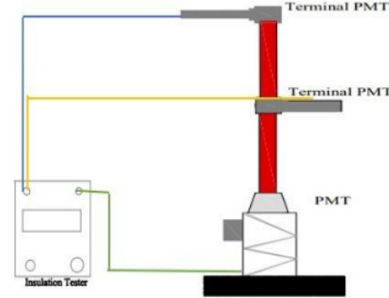
Gambar 7. Pengujian Tahanan Isolasi.
