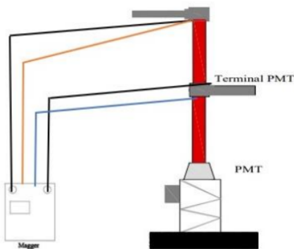
Gambar 8. Pengujian Tahanan Kontak.
