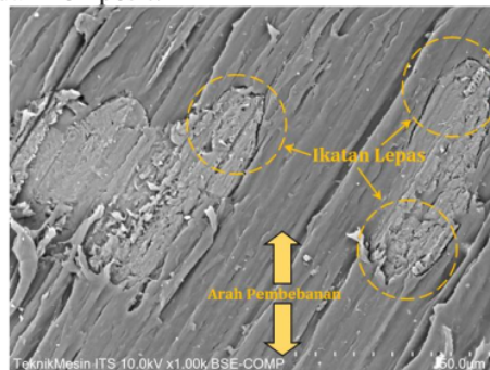
Gambar 11: Foto Mikro Antarmuka Samping Komposit Volume STK 7% Ukuran 250-300 mesh
