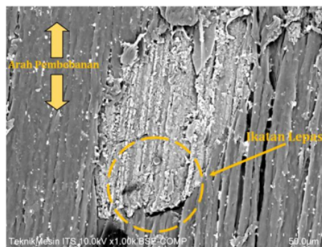
Gambar 12: Foto Mikro Antarmuka Samping Komposit Volume STK 13% Ukuran 100-150 mesh
