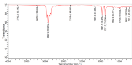
Gambar 4: Hasil FTIR Komposit Volume STK 7% Ukuran 100-150 mesh.
