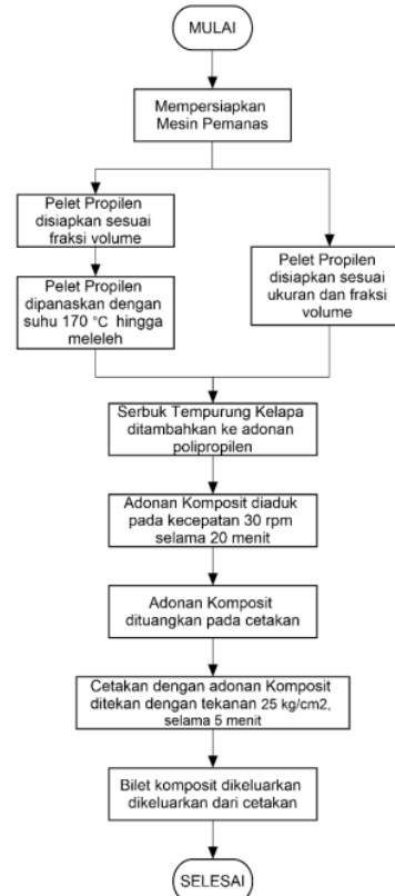
Gambar 1: Diagram Alir Pembuatan Komposit
