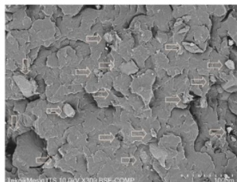
Gambar 8: Foto Mikro Komposit Volume STK 7% Ukuran 100-150 mesh. (Panah menunjukkan posisi penguat)
