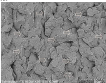
Gambar 7: Foto Mikro Komposit Volume STK 13% Ukuran 250-300 mesh. (Panah menunjukkan posisi penguat)
