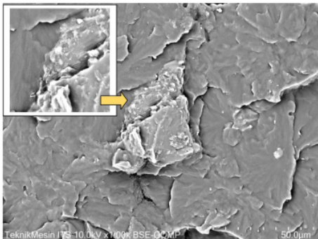
Gambar 10: Foto Mikro Antarmuka Melintang Komposit Volume STK 7% Ukuran 100-150 mesh
