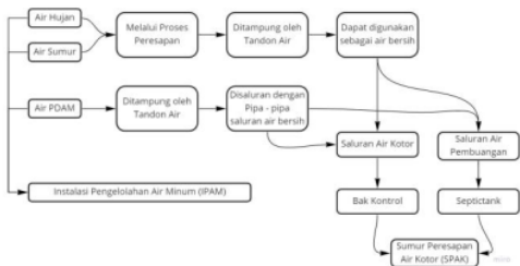
Gambar 5.3 Bagan Konsep Utilitas Air bersih & Air Kotor Sumber : Data pribadi
