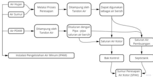
Gambar 5.1 Bagan Konsep Drainase Air Sumber : Analisa Penulis, 2022
