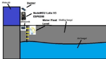
Gambar 3 Penerapan alat di lokasi
