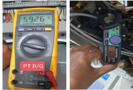
Gambar 4.7 Hasil Pengukuran Tegangan dan Arus
