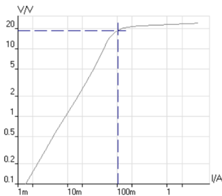
Gambar 4.5 Hasil Pengujian Excitasi CT
