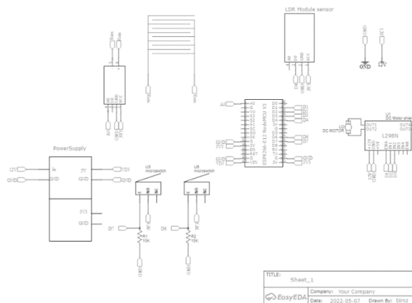
Gambar 3. 2 Skematik Alat
