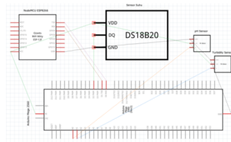
Gambar 4. Rangkaian Alat Pengukuran
