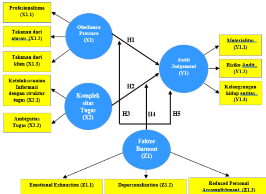
Gambar 1. Kerangka Konseptual
