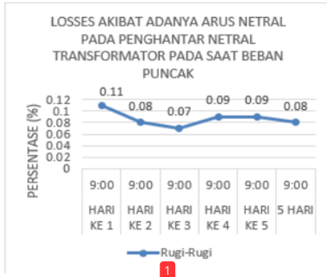
Gambar 10. Grafik Losses Akibat Adanya Arus Netral Di Penghantar Netral Trafo Saat Beban Puncak
