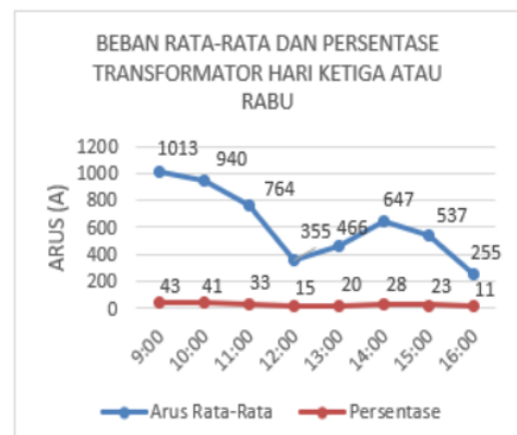
Gambar 5. Grafik Beban Rata-Rata & Presentase Hari Rabu
