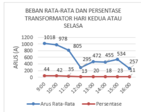
Gambar 4. Grafik Beban Rata-Rata & Presentase Hari Selasa
