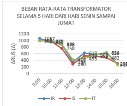
Gambar 8. Grafik Beban Rata-Rata & Persentase Selama 5 hari
