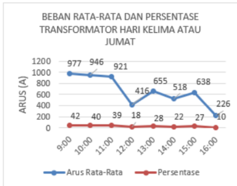
Gambar 7. Grafik Beban Rata-Rata & Presentase Hari Jumat
