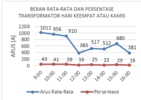
Gambar 6. Grafik Beban Rata-Rata & Presentase Hari Kamis
