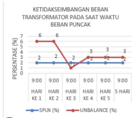
Gambar 9. Grafik Ketidakseimbangan Beban Saat Waktu Beban Puncak
