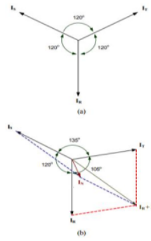
Gambar 1. Ketidakseimbangan Beban
