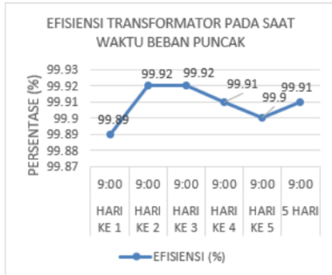
Gambar 11. Grafik Efisiensi Beban Puncak
