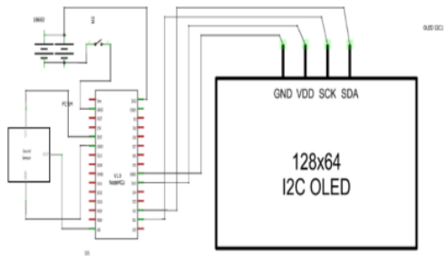
Gambar 3.2 Skematik Alat
