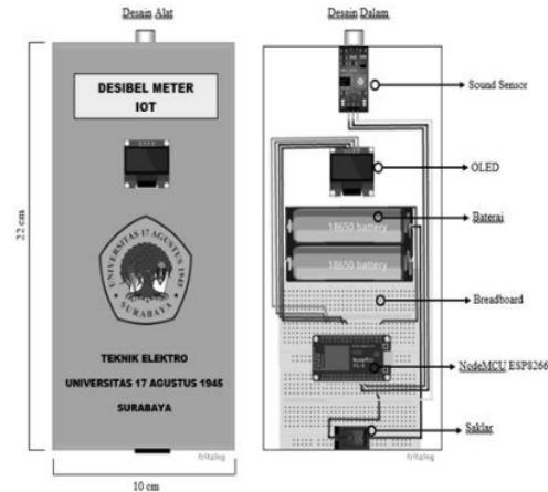
Gambar 3.4 Desain Alat
