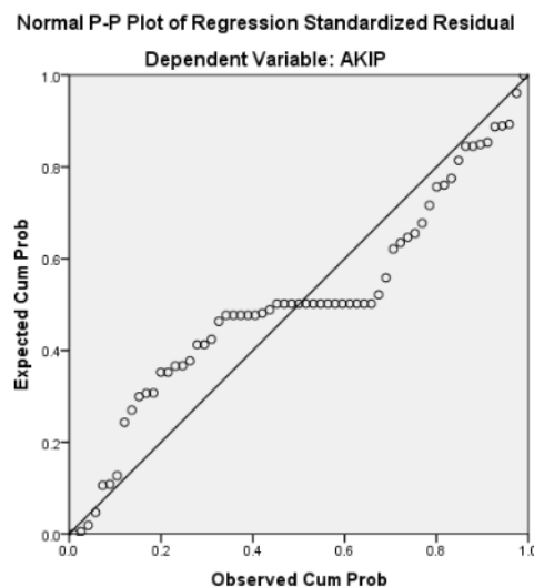
Gambar 4.1 Uji Normalitas dengan Grafik Normal P-Plot
