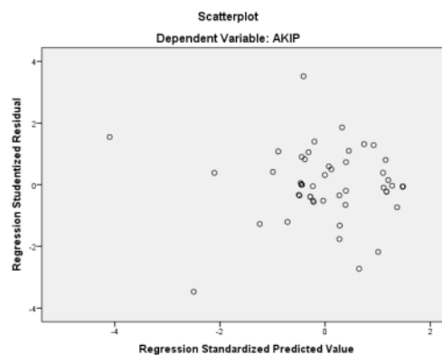
Gambar 4.2 Uji Heteroskedastisitas dengan Grafik Plot (Scatterplot)
