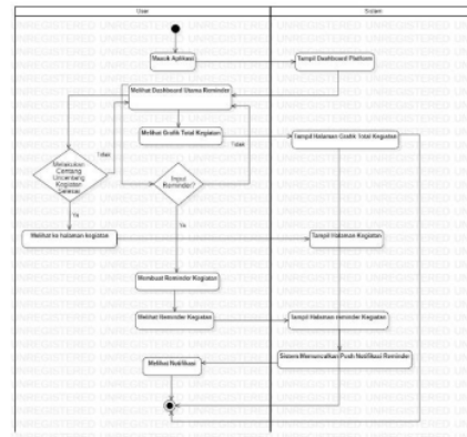
Gambar 4. Diagram Activity Membuat Reminder
