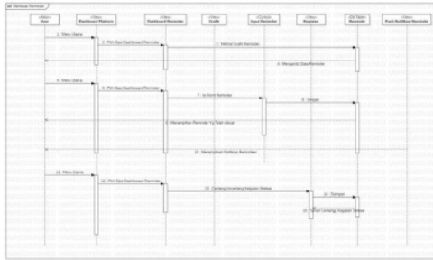
Gambar 5. Diagram Sequence Membuat Reminder
