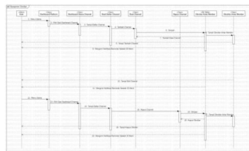
Gambar 9. Diagram Sequence Mengelola Percakapan
