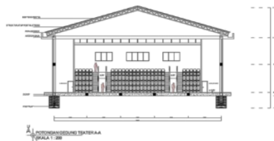
Gambar12 Potongan Masa Utama
