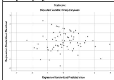
Gambar 2 Uji Heterokedastisitas
