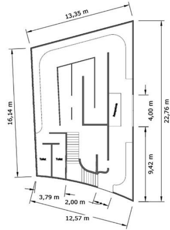
Galeri Lt 1 Skala : 1:200
