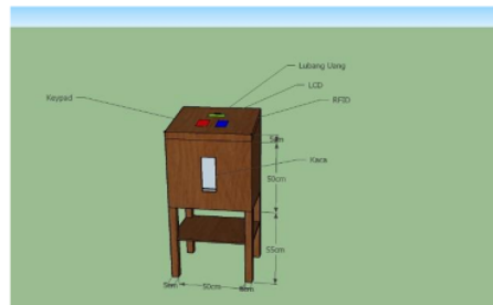
Gambar 2. 1 Perancangan Fisik Kotak Amal
