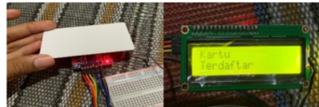
Gambar 3. 2 Pengujian RFID
