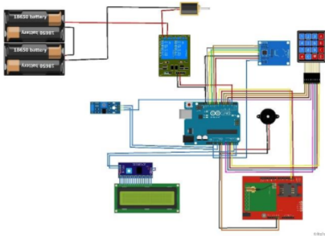
Gambar 2.5 Rangkaian Seluruh Sistem
