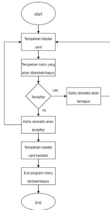
Gambar 2. 4 Flowchart Menu Hapus dan Tambah
