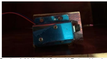
Gambar 3.26 Kondisi Solenoid Terkunci kembali
