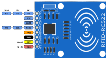
Gambar 1. 5 Modul RFID
