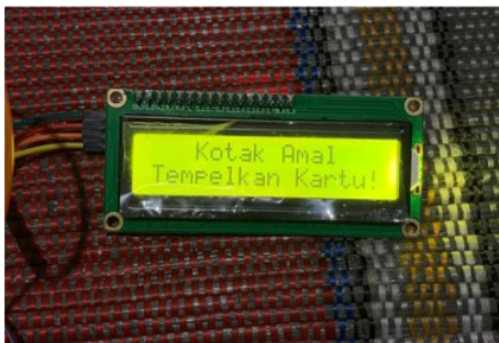
Gambar 3. 6 Pengujian LCD
