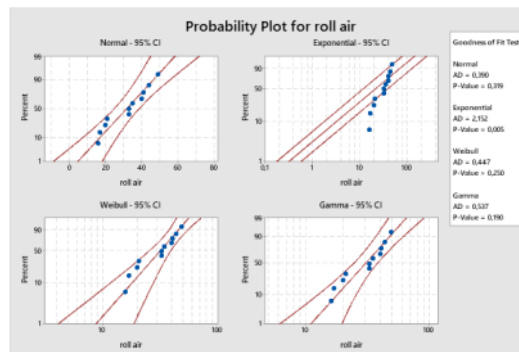
Gambar 2 Hasil Pengujian Komponen Roll Air
