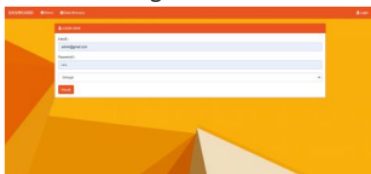
Gambar 10. Halaman login
