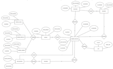
Gambar 6.ERD
