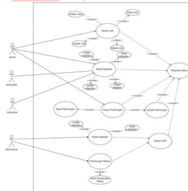
Gambar 3. Use Case Skenario
