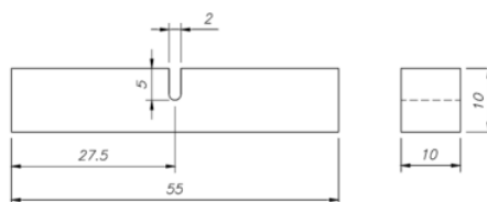
Gambar 12. Dimensi Spesimen Uji Impact
