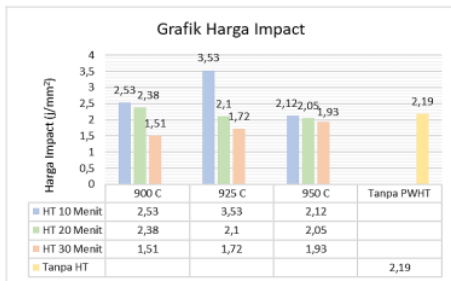
Gambar 14. Grafik Harga Impact
