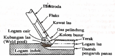
Gambar 1. Skema Las SMAW
