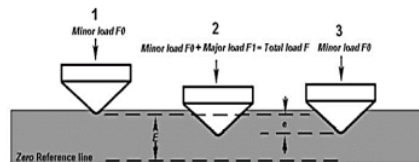
Gambar 4. Skema Uji Kekerasan Rockwell C
