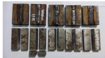
Gambar 9. Spesimen Pengelasan
