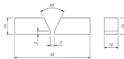
Gambar 7. Dimensi Kampuh Las
