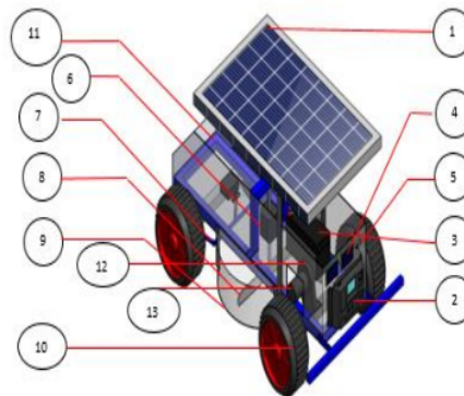
Gambar 6 Rancangan Potong Rumpit Elektrik Tenaga Surya
