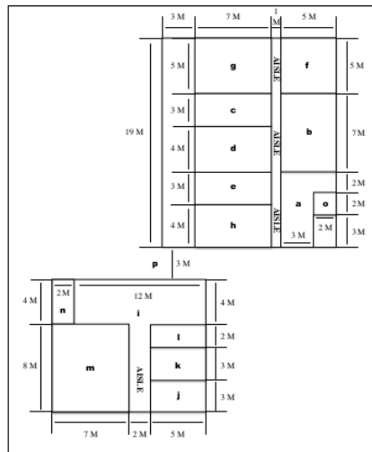
Gambar 8. Denah Baru Skenario Dua
