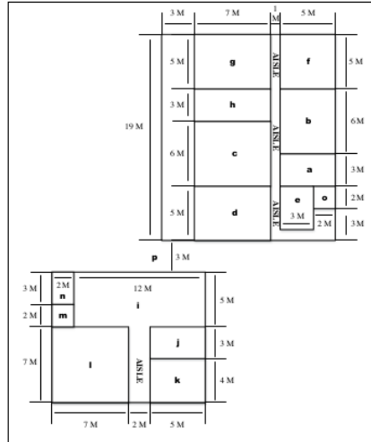
Gambar 7. Denah Baru Skenario Satu
