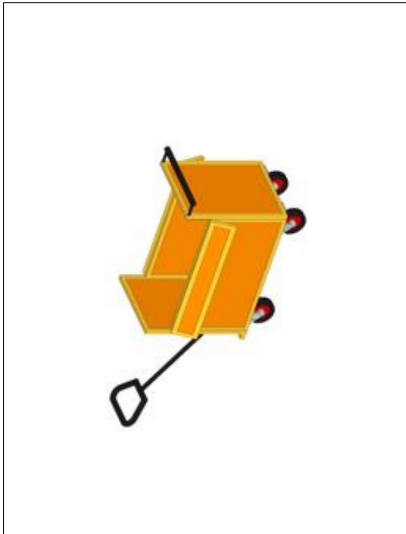
Lampiran 2 Gambar 3D rancangan alat angkut posisi terbuka
