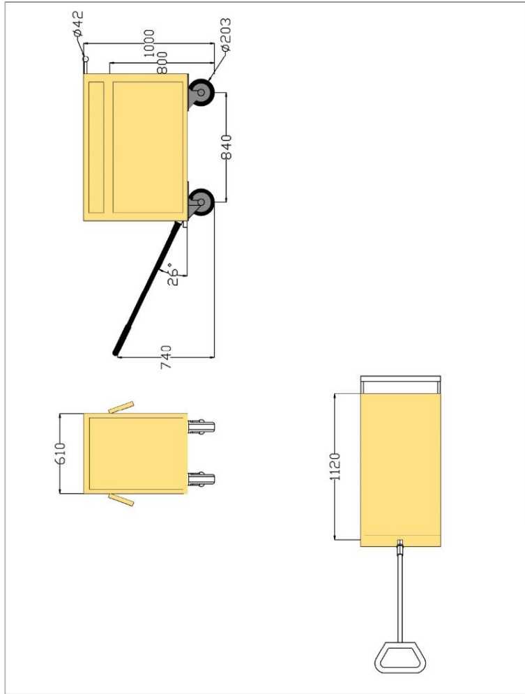
Lampiran 3 Gambar 2D rancangan alat angkut posisi tertutup
