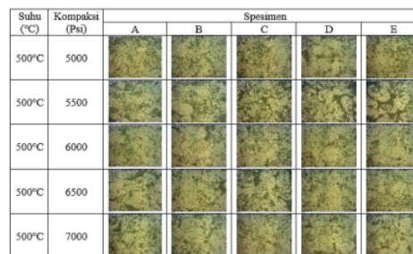
Gambar 12. Hasil uji struktur mikro Al-Ti komposisi 6% suhu 500°C
