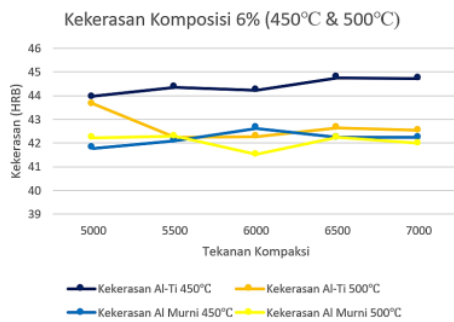
Gambar 9. Grafik hasil uji kekerasan komposisi Ti 6%
