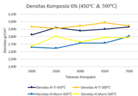
Gambar 8. Grafik hasil uji densitas komposisi Ti 6%
