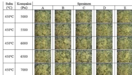
Gambar 11. Hasil uji struktur mikro Al-Ti komposisi 6% suhu 450°C
