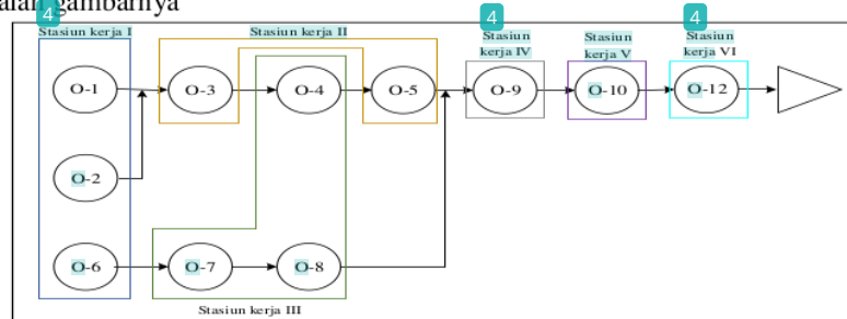
Gambar 4 Precedence Diagram dan Stasiun Kerja Kondisi Aktual
