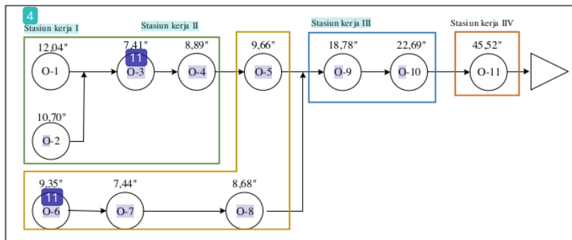
Gambar 5 SK kondisi Usulan Penambahan TK sesudah LB
