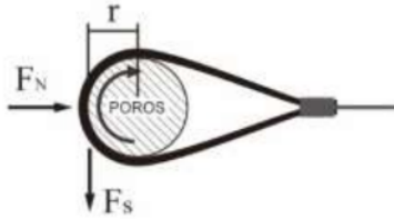
Gambar 16 Bidang Gesek Pada Poros.
