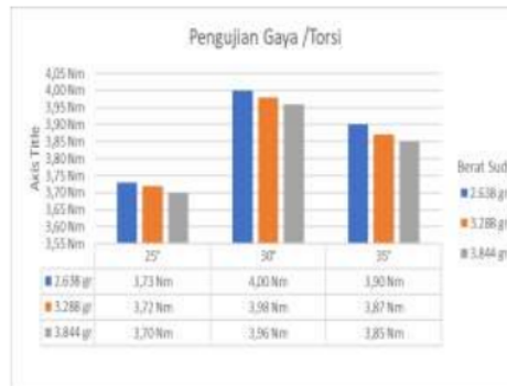
Gambar 14 Hasil pengujian torsi turbin angin dengan kecepatan 2.0 m/s.
