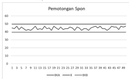
Gambar 1. Grafik keseragaman data pemotongan spon
