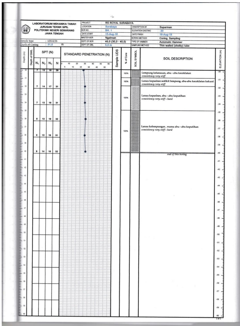
10. Data Tanah Proyek Rs. Royal (Sumber : Data Proyek, 2021)
