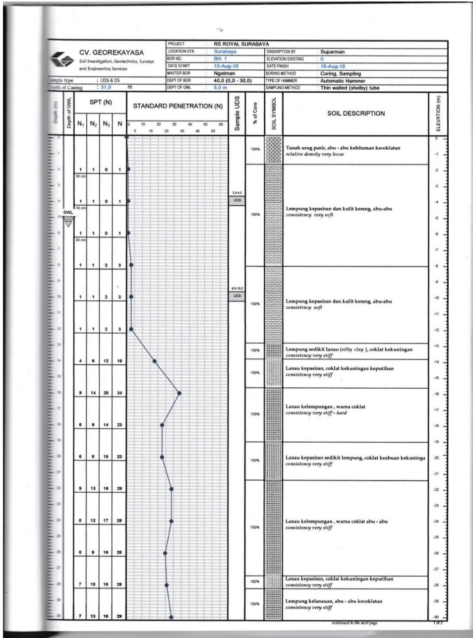
9. Data Tanah Proyek Rs. Royal (Sumber : Data Proyek, 2021)
