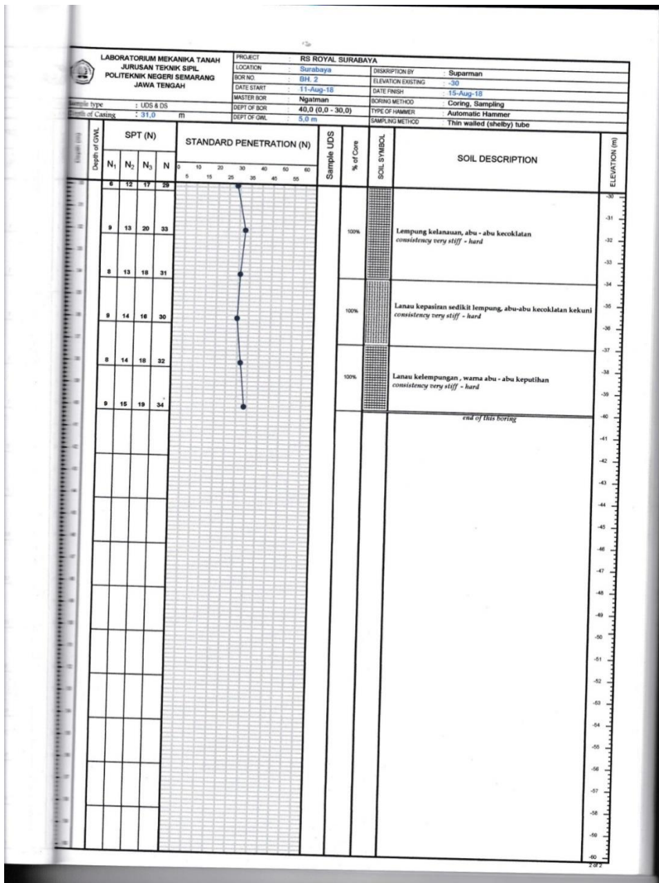
11. Data Tanah Proyek Rs. Royal (Sumber : Data Proyek, 2021)
