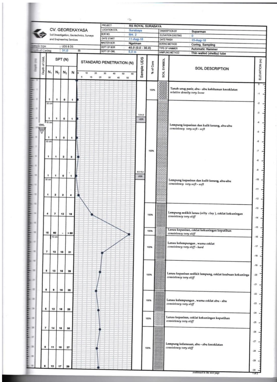
8. Data Tanah Proyek Rs. Royal (Sumber : Data Proyek, 2021)
