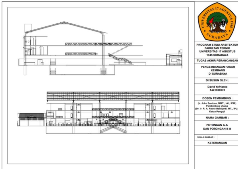
Gambar 74 Potongan A-A B-B
