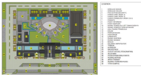
Gambar 10. Site Plan Sumber: Data Penulis, 2022
