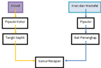
Gambar 12. jaringan air kotor
