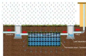
Gambar 11. Konsep penampungan air
