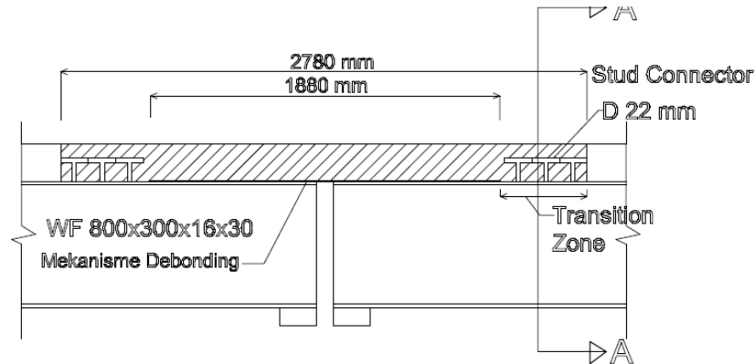
Gambar 3.5 Link Slab memanjang pada bentang 18 m
