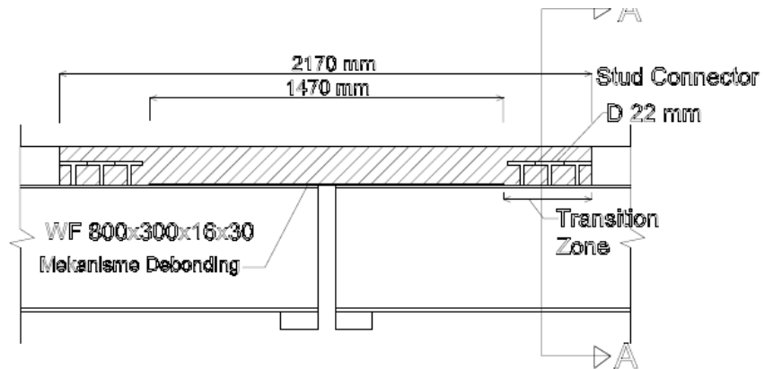
Gambar 3.3 Link Slab memanjang pada bentang 14 m
