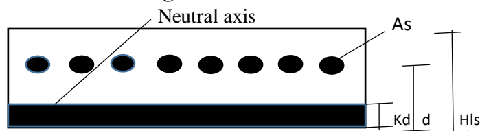
Gambar 3.1 Ilustrasi penentuan luasan tulangan Link Slab Bentang 14 m Untuk perencanaan link slab jembatan ini menggunakan data sebagai berikut :
