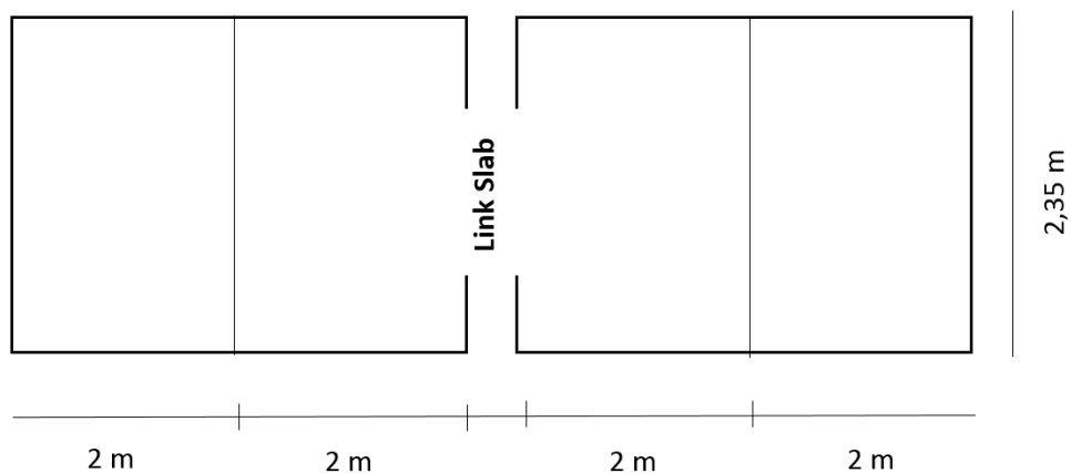
Gambar 3.2 Detail Link Slab tampak atas
