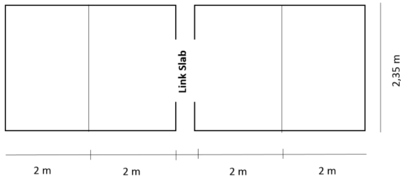
Gambar 3.2 Detail Link Slab tampak atas
