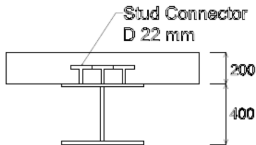
Gambar 3.4 Link Slab melintang potongan A-A pada bentang 14 m
