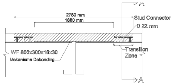
Gambar 3.5 Link Slab memanjang pada bentang 18 m
