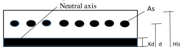
Gambar 3.1 Ilustrasi penentuan luasan tulangan Link Slab Bentang 14 m
