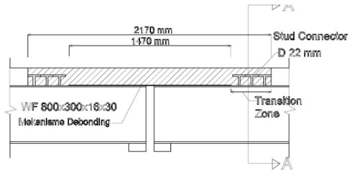
Gambar 3.3 Link Slab memanjang pada bentang 14 m
