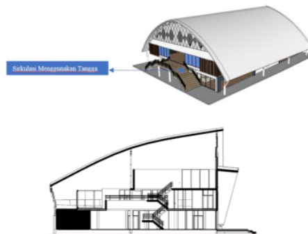
Gambar 14. Konsep Sirkulasi
