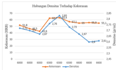
Gambar 14. Hubungan Densitas dan Kekerasan
