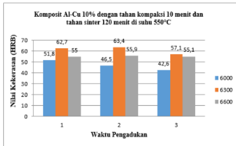
Gambar 12. Pengaruh Variasi Waktu Pengadukan Terhadap Kekerasan
