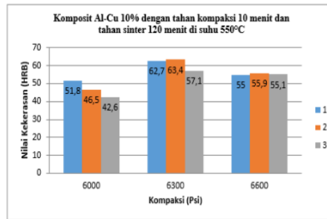
Gambar 11. Pengaruh Variasi Tekanan Kompaksi Terhadap Kekerasan
