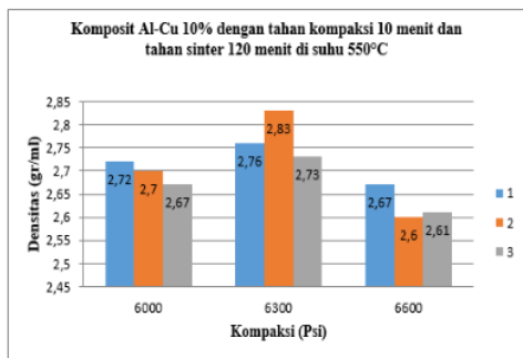
Gambar 13. Pengaruh Variasi Tekanan Kompaksi Terhadap Densitas
