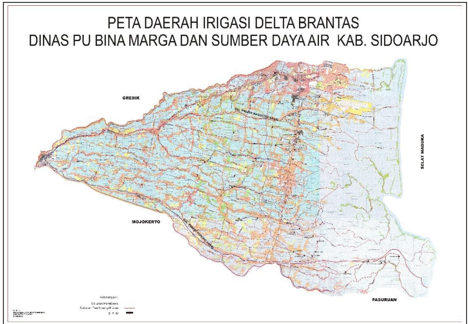
Gambar 1 Peta Irigasi.
