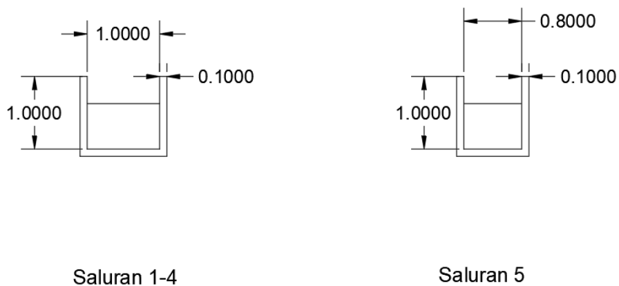
Gambar 10. Hasil Evaluasi Dimensi saluran kawasan perum Kepuh Permai
