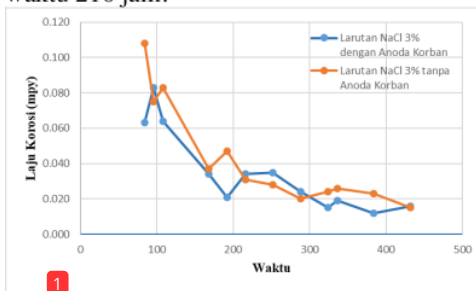
Gambar 4. 11 Grafik Laju Korosi Larutan NaCl 3%
