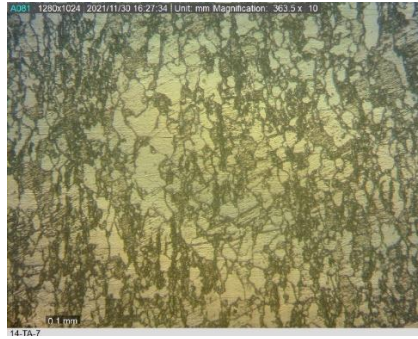
Struktur mikro larutan NaCl 7% tanpa Anoda
