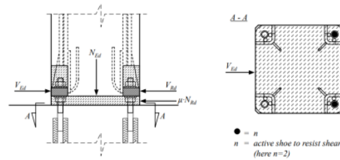
Gambar 2. Konfigurasi Sepatu Kolom
