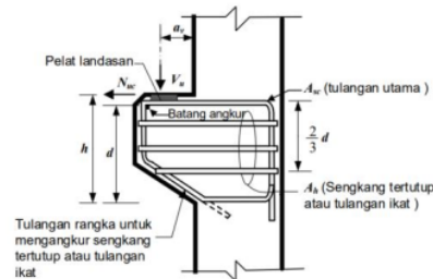
Gambar 1. Penampang Konsol Pendek
