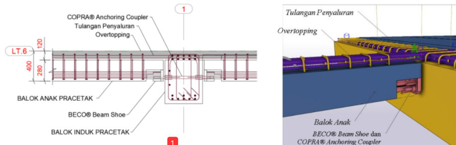
Gambar 7. Sambungan Balok Induk - Balok Anak
