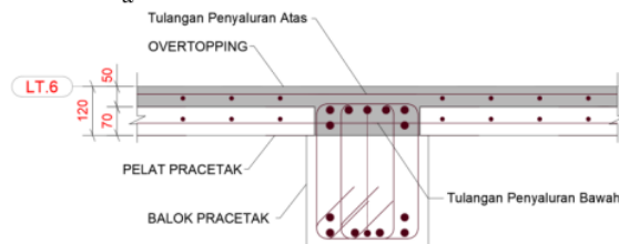
Gambar 8. Sambungan Pelat - Balok Anak
