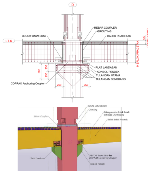
Gambar 6. Sambungan Kolom - Kolom dan Balok Induk – Kolom
