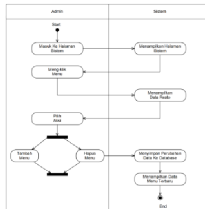
Gambar 7. Diagram Aktivitas Kelola Menu
