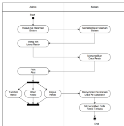
Gambar 6. Diagram Aktivitas Kelola Resto
