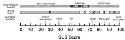
Gambar 14. SUS Score
