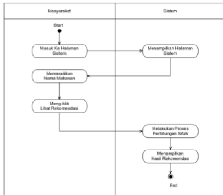
Gambar 9. Diagram Aktivitas Cari Makanan
