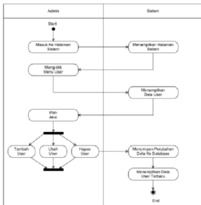
Gambar 5. Diagram Aktivitas Kelola User
