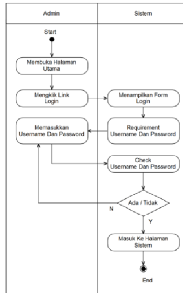
Gambar 4. Diagram Aktivitas Login
