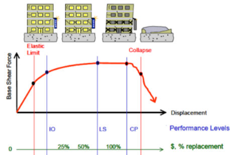
Gambar 2. Ilustrasi Perancangan Berbasis Kinerja (Sumber: Kajian Penulis)
