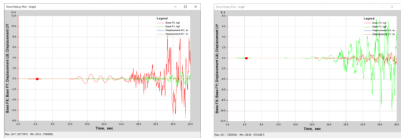
Gambar 7. Contoh Plot Base Shear Reaction Akibat Beban Gempa NLTHA (Sumber: Kajian Penulis)
