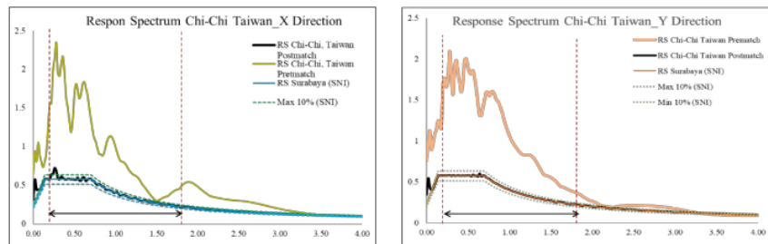
Gambar 4. Contoh Grafik Elastic Design Spectrum (EDS) (Sumber: Kajian Penulis)
